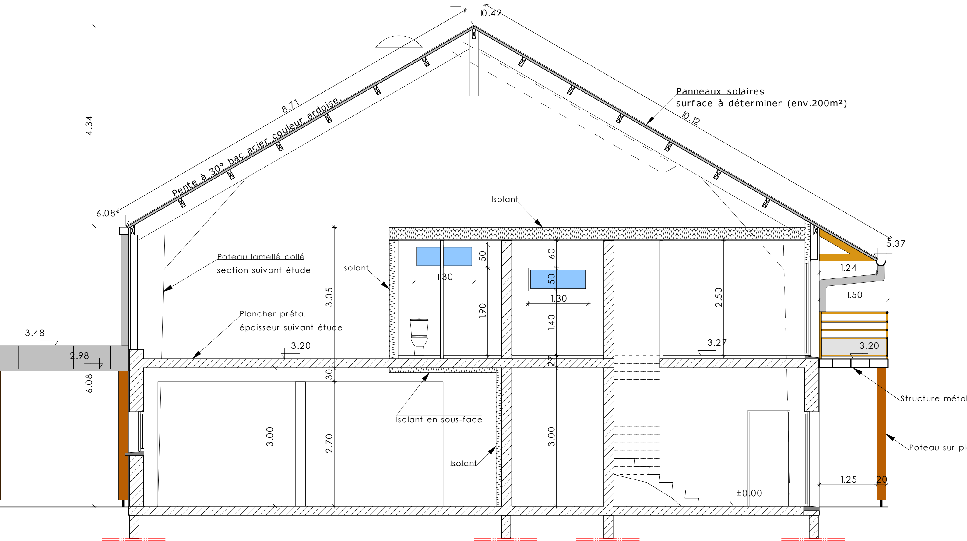
Coupe au 1/50°. Avril 2010.
