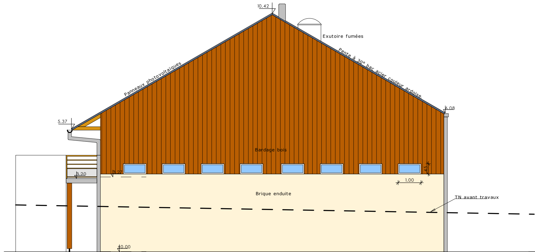
Façade est
