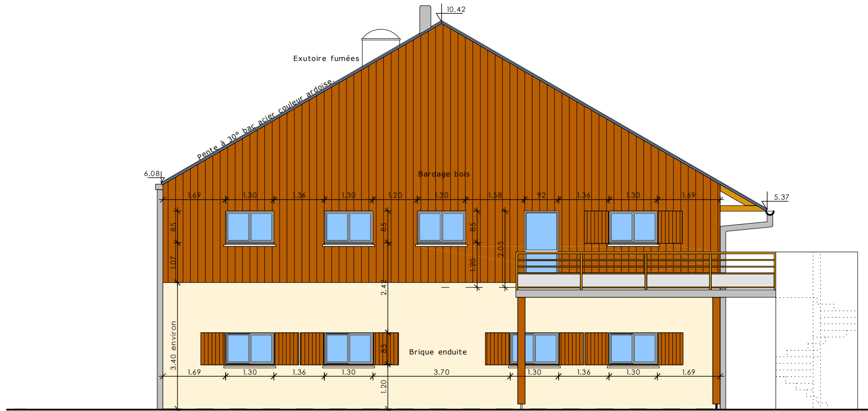
Façade ouest
