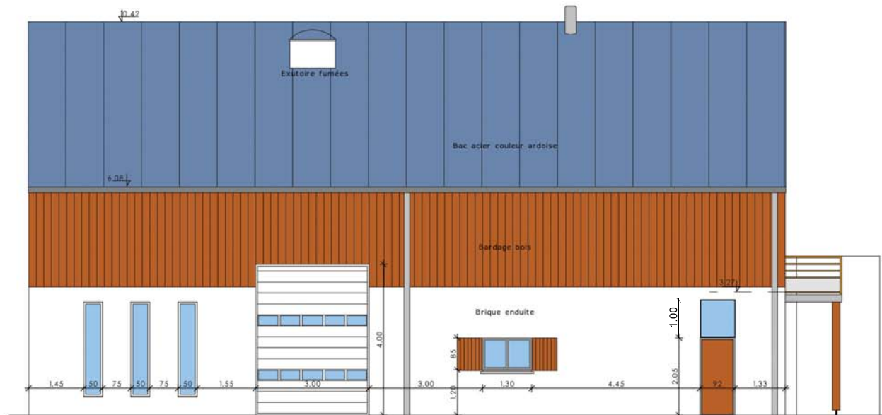
Façade nord
